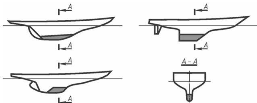
Рис. 3.5.1-1. Яхта с классическим фальшкилем
